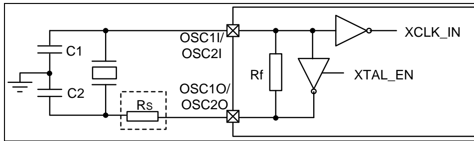
图 2-8 XTAL 振荡器电路结构示意图
