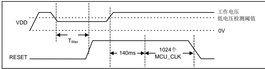
图 2-4 掉电复位时序示意图
