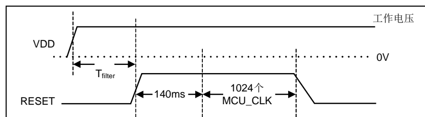
图 2-3 上电复位时序示意图
