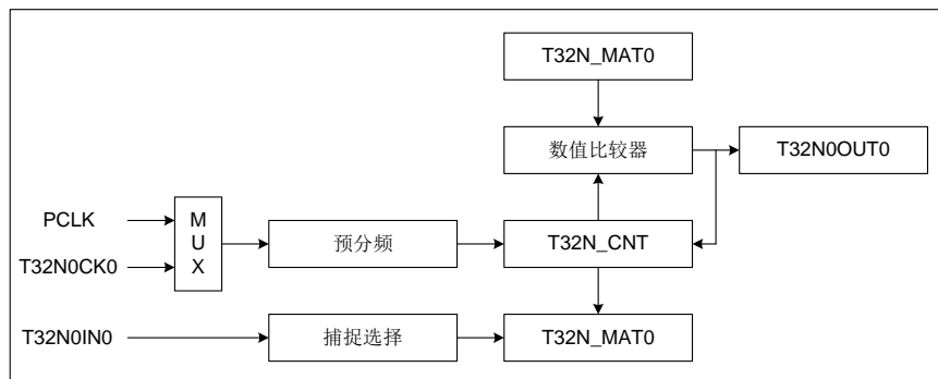
图 5-7 T32N0 电路结构框图
