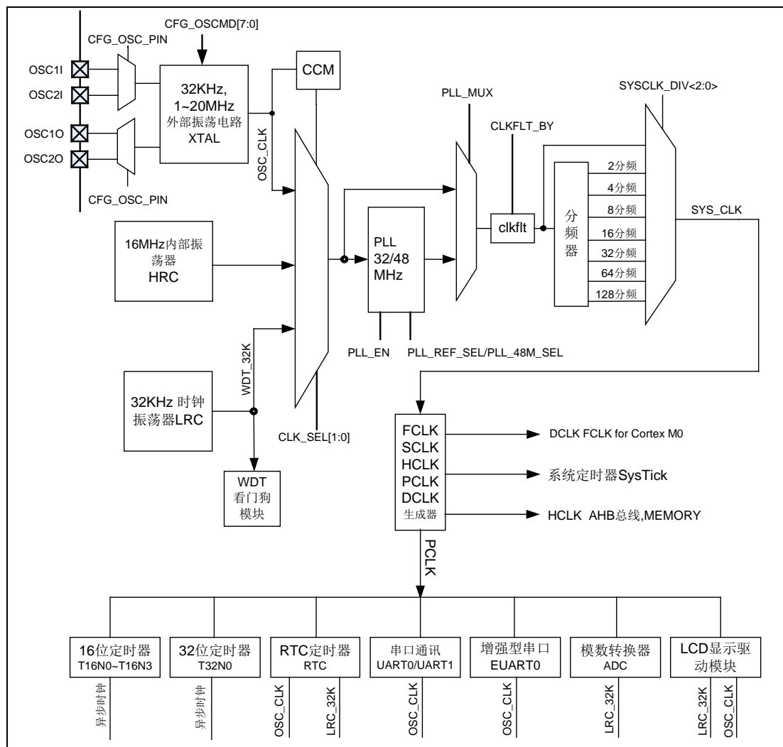
图 2-7 系统时钟电路结构框图
