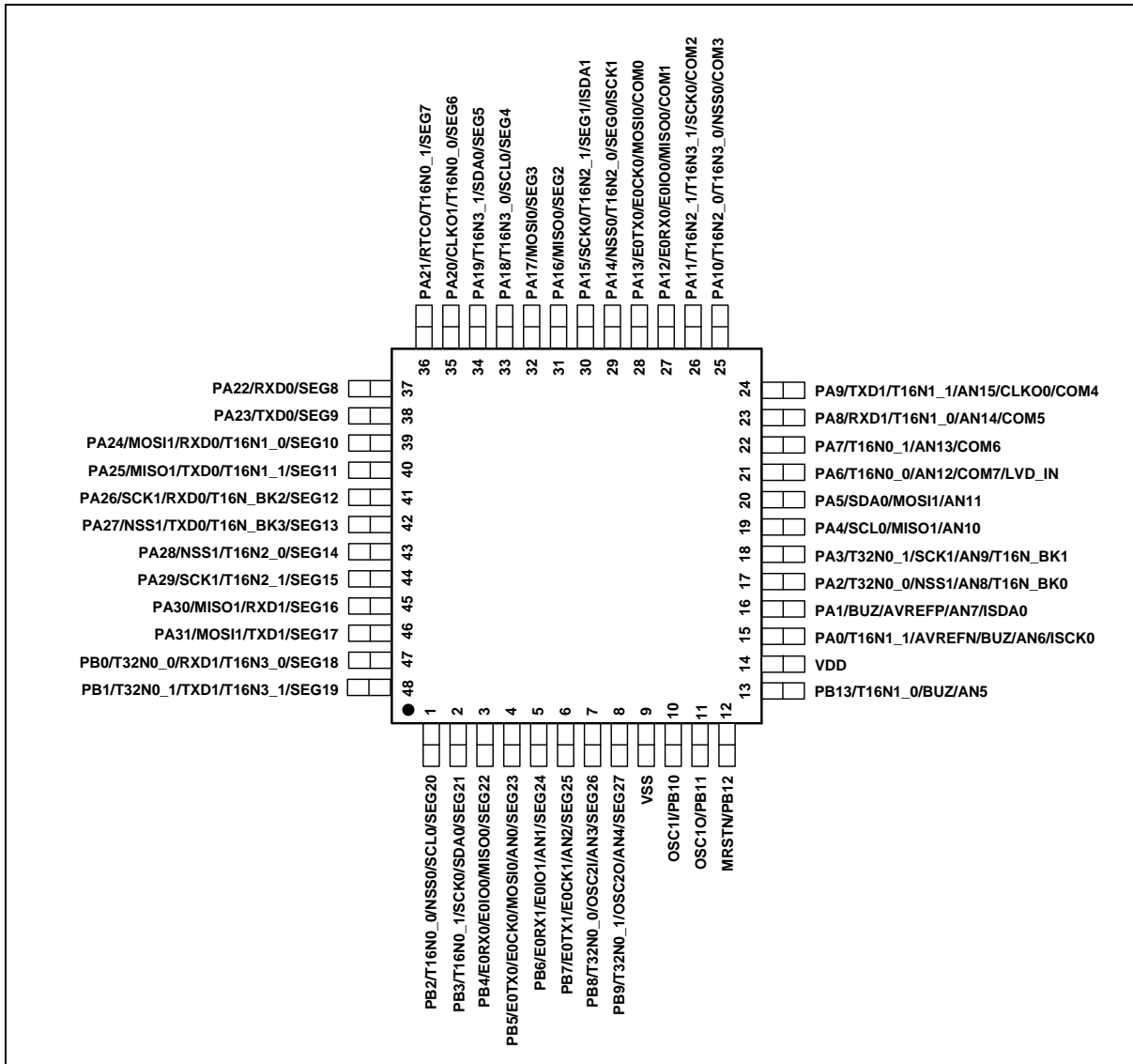
图 1-2 LQFP48 封装顶视图
