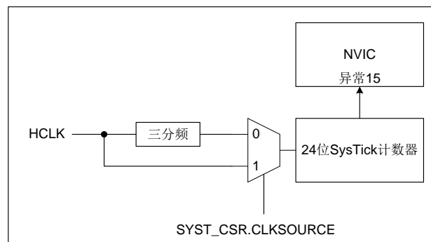
图 2-9 系统定时器框图
