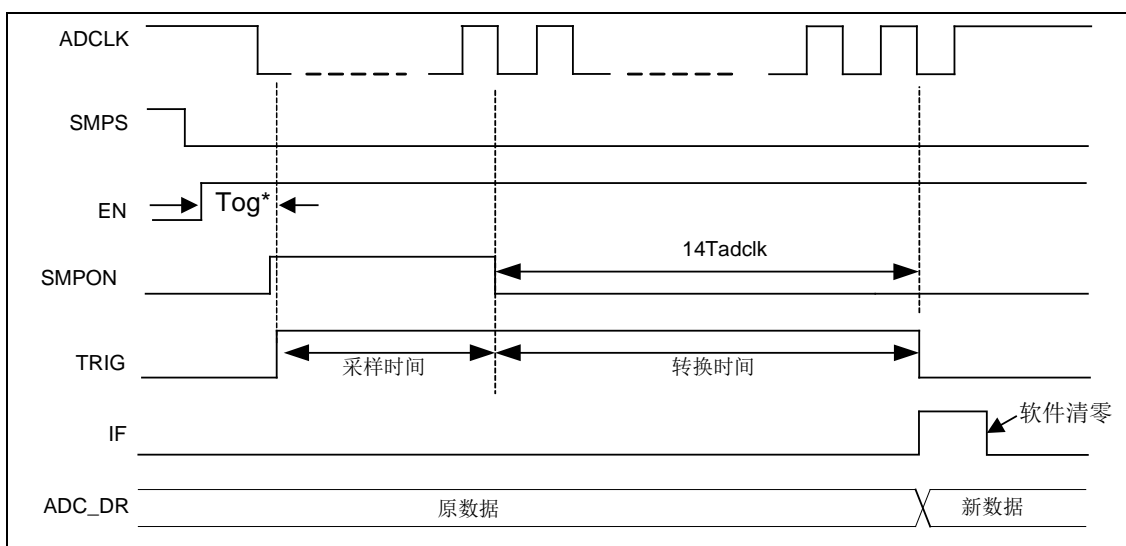
图 5-50 ADC 数据转换时序示意图（ADC_CON1 寄存器的 SMPS=0，软件控制采样）
