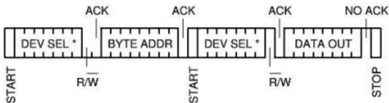
图 14 I 2 C 读取时序图
