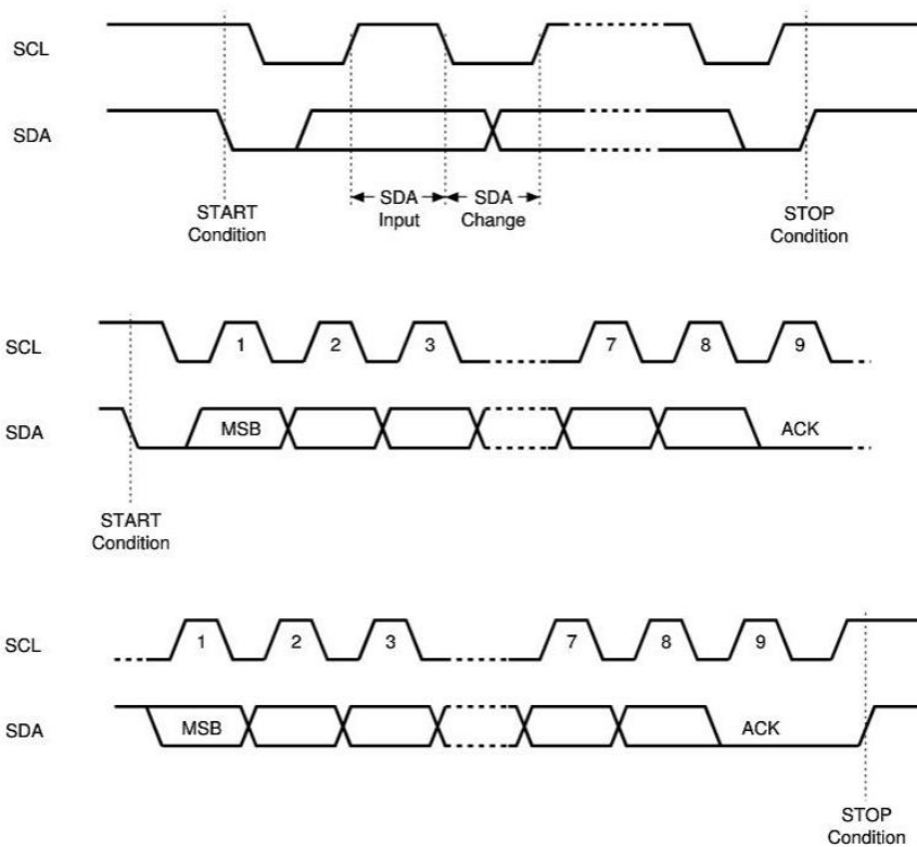
图 13 I 2 C 通信协议
