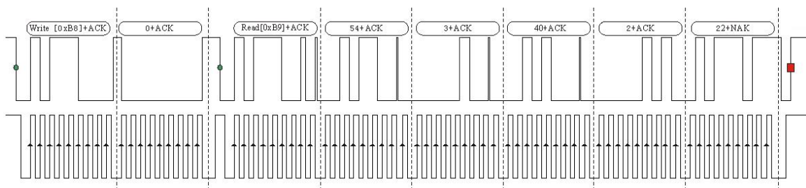
图 15 参考时序图
