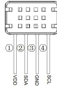
图 4: DHT12 接线图
