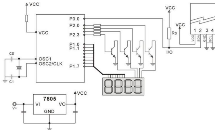
图 19 典型电路图
