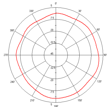
AN1603-868 E-Plane
