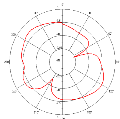
AN1603-868 E-Plane
