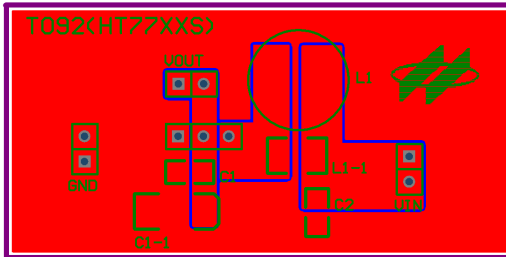
Top Layer
