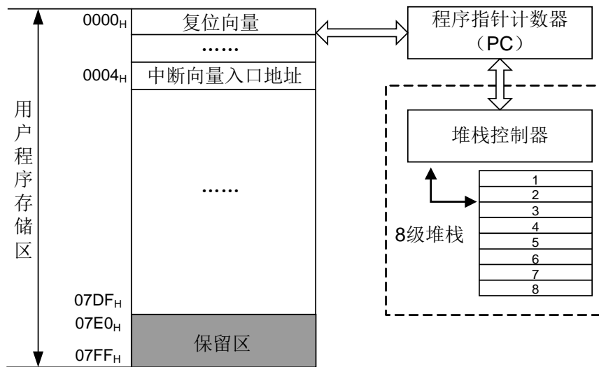
图 3-1 HR7P167 程序区地址映射和堆栈示意图
