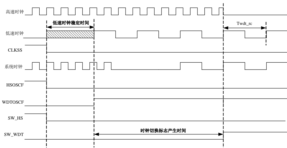
图 6-5 INTOSCL 时钟切换到 HS/XT/RC/INTOSCH 时钟时序图
