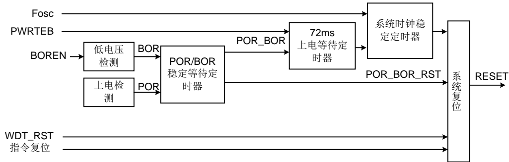
图 6-10 芯片复位原理图
