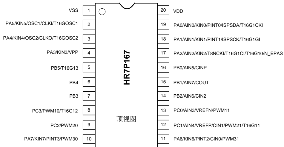
图 1-4 DIP20/SOP20/SSOP20 顶视图
