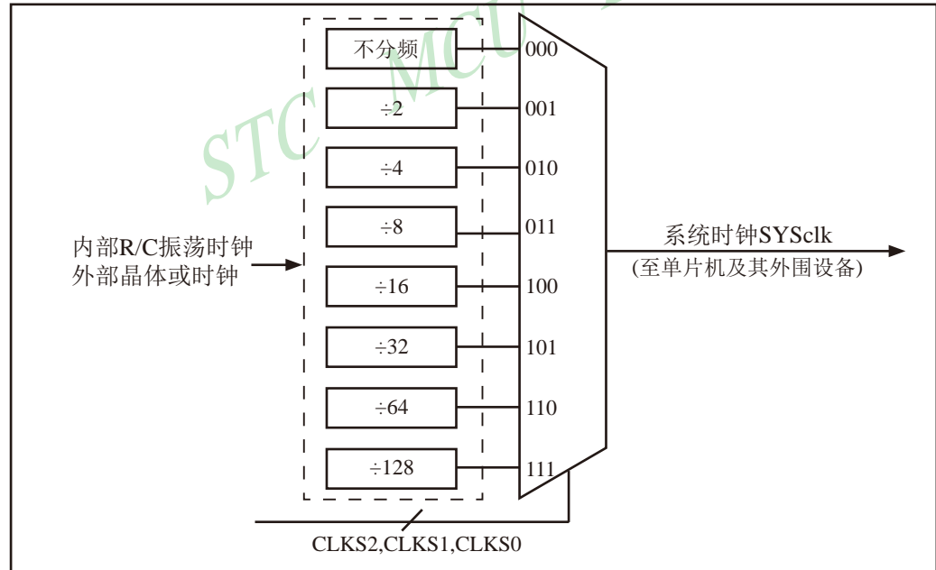
时钟结构
