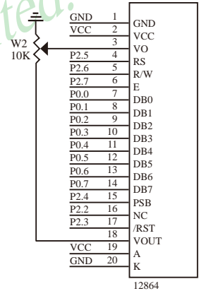
液晶模块 12864接口插座 R82、R83调整LCD背光亮度
