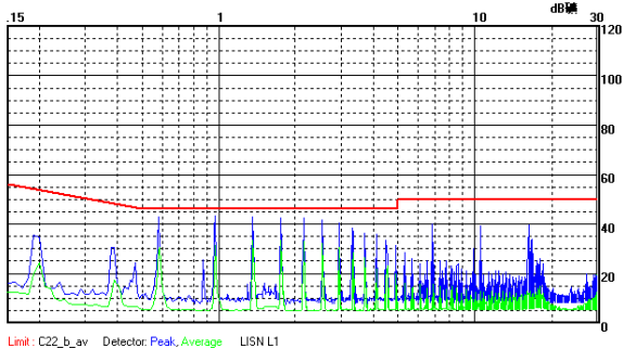
A2415S-1WR2 传导骚扰 Class B 测试效果图 (正线)
