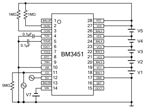
测试电路 4
