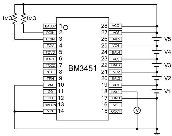
测试电路 5
