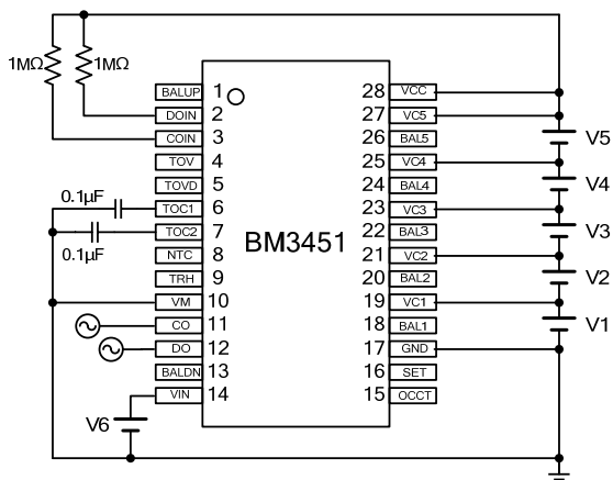
测试电路 3
