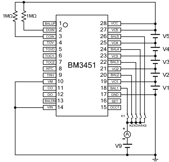
测试电路 8
