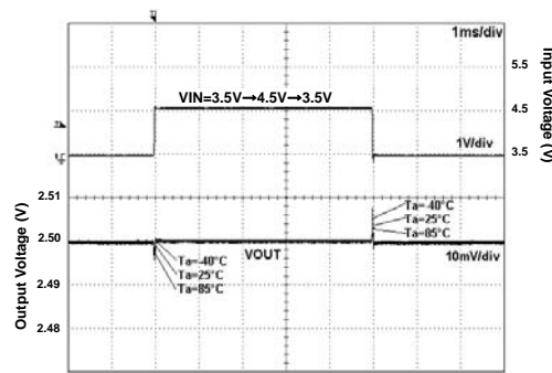
Fig 128. VIN Response
