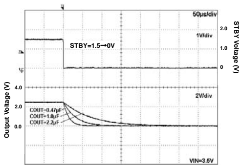
Fig 127. Discharge Time
