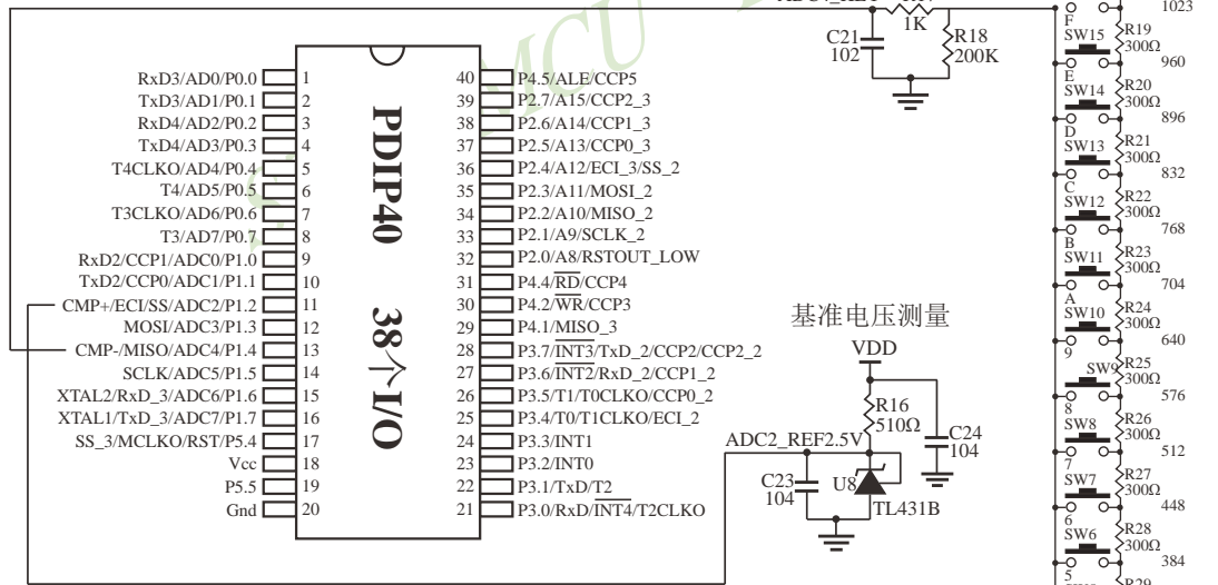
16个ADC按键
