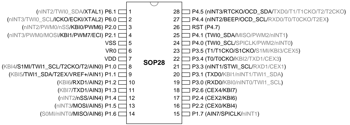
图 5-2. MA82G5BxxAS28 顶视图
