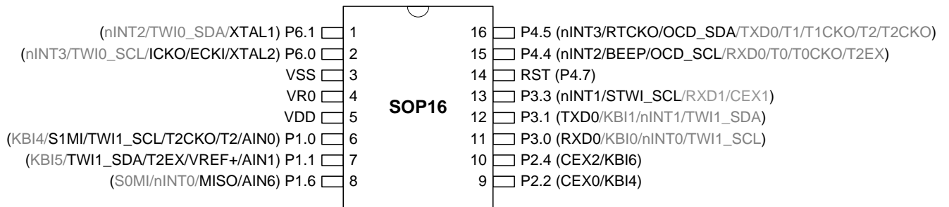
图 5-4. MA82G5BxxAS16 顶视图
