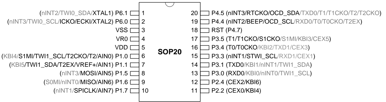
图 5-3. MA82G5BxxAS20 顶视图
