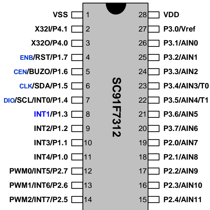
SC91F7312管脚配置图
