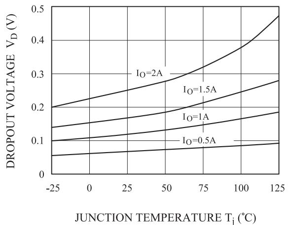
Fig.9 T_j - V_D
