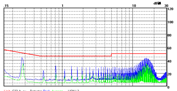
WRF1205S-3WR2 传导骚扰 Class B 测试效果图 (负线)
