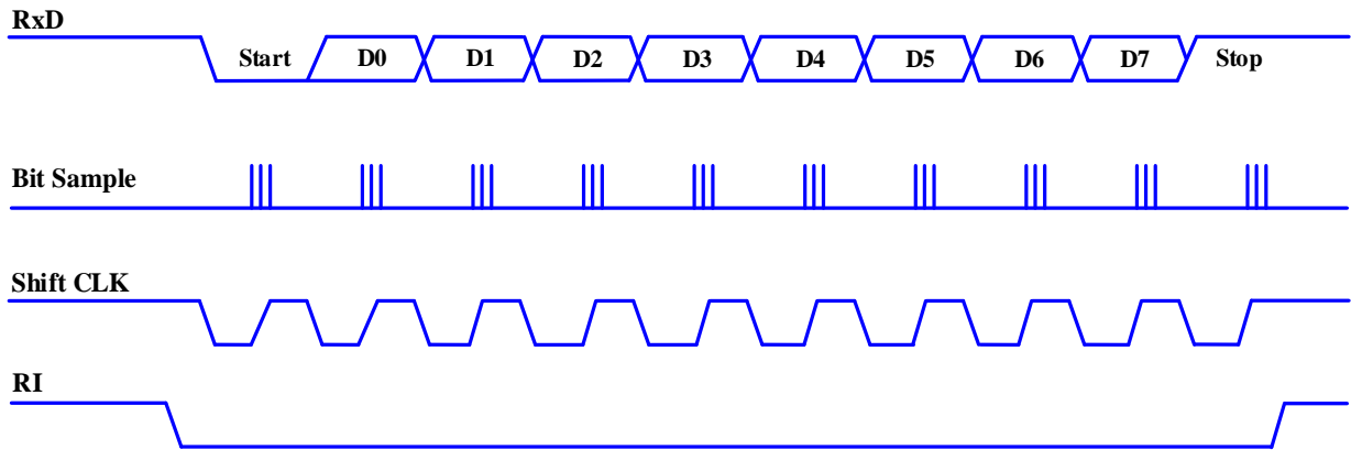
模式1:接收时序图
