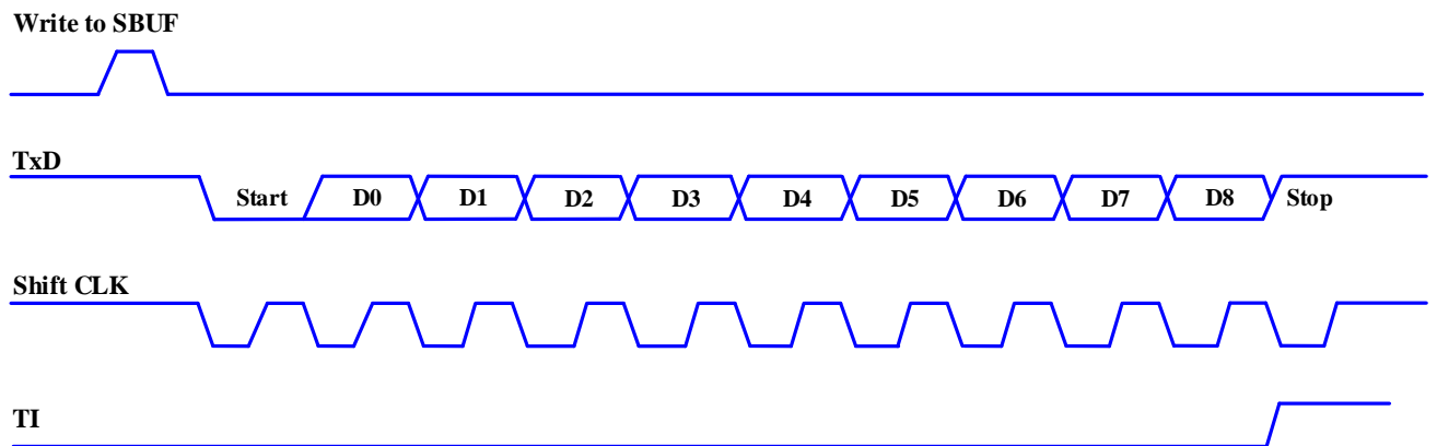
模式3:发送时序图
