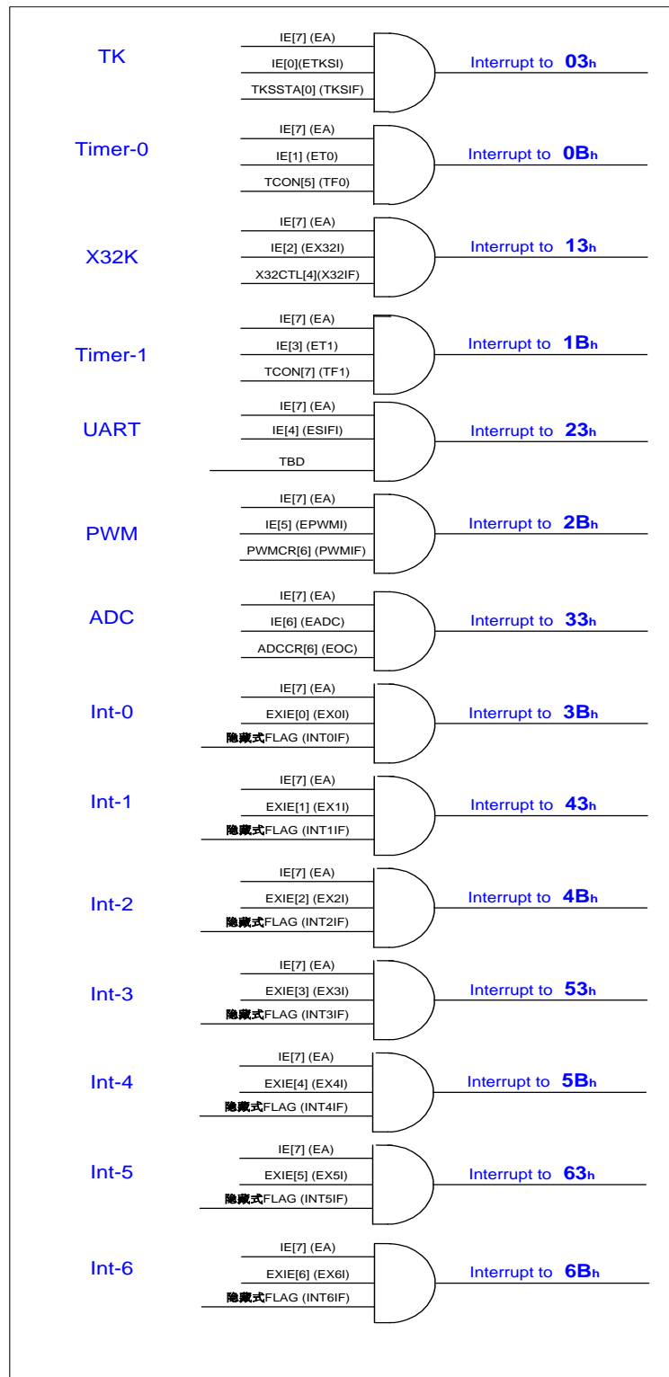
SC91F844中断结构和向量
