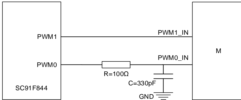
PWM0输出端增加RC延时电路
