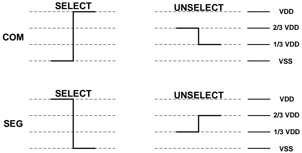
1/3Bias LCD 应用中 COM 和 SEG 的波形图:
