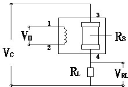
图 2： MP503 测试电路
