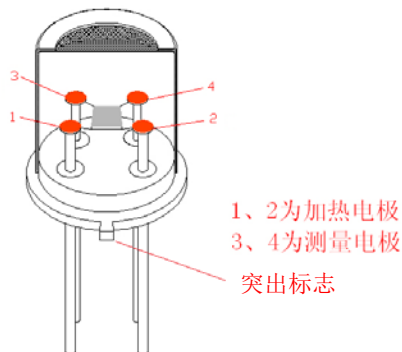
图 8： 管脚示意图
