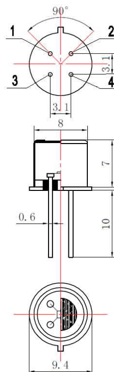
图 1: 传感器结构图
