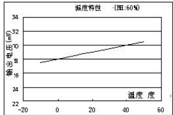
图6：灵敏度温度特性曲线
