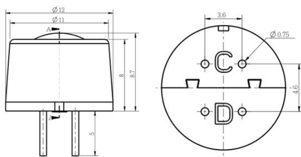
图 1: 元件外形结构
