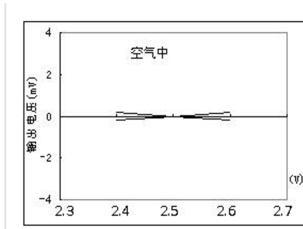
图 9：零点电源波动特性曲线
