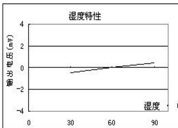
图7：零点湿度特性曲线
