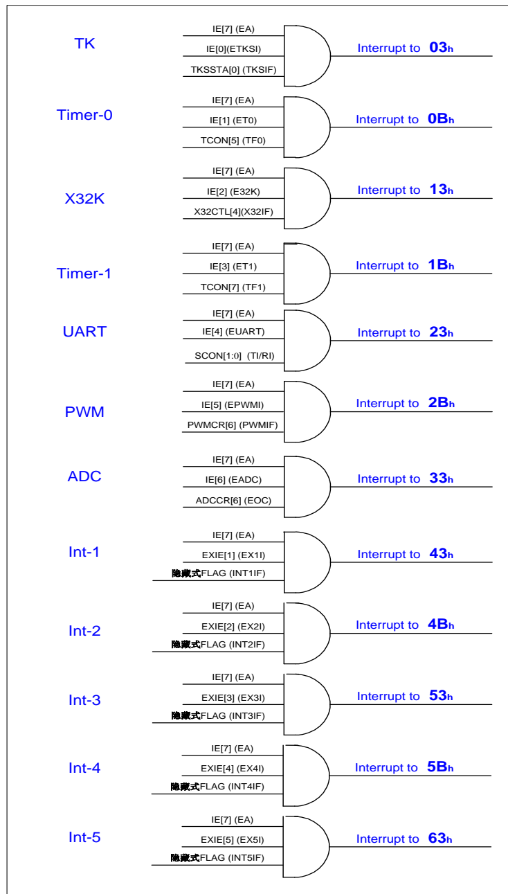
SC91F846中断结构和向量
