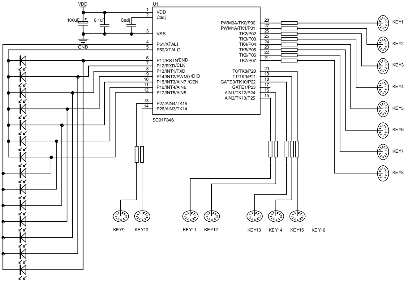
应用电路 2: LED 显示和 TK 不共用 (仅供参考)
