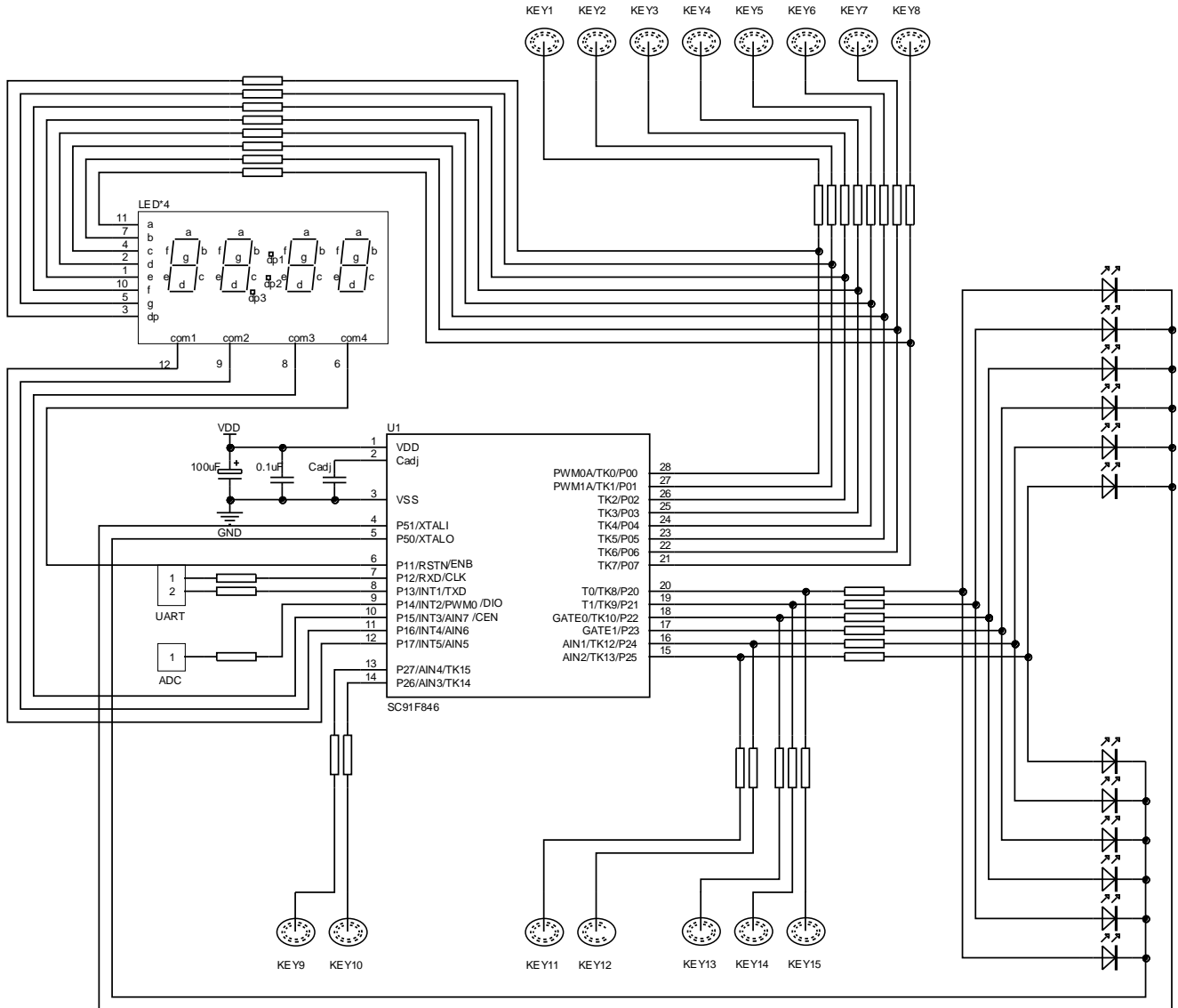
应用电路 1: LED 显示和 TK 共用 (仅供参考)
